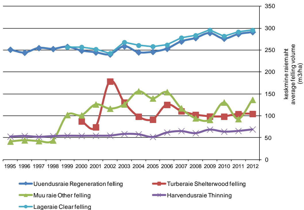
Joonis 3.3.3.2 Riigimetsamaa keskmine raiemaht hektari kohta aastail 1993–2012 (m 3 /ha) Figure 3.3.3.2 Average felling volume per hectare in state forest in 1993–2012 (m 3 /ha)
