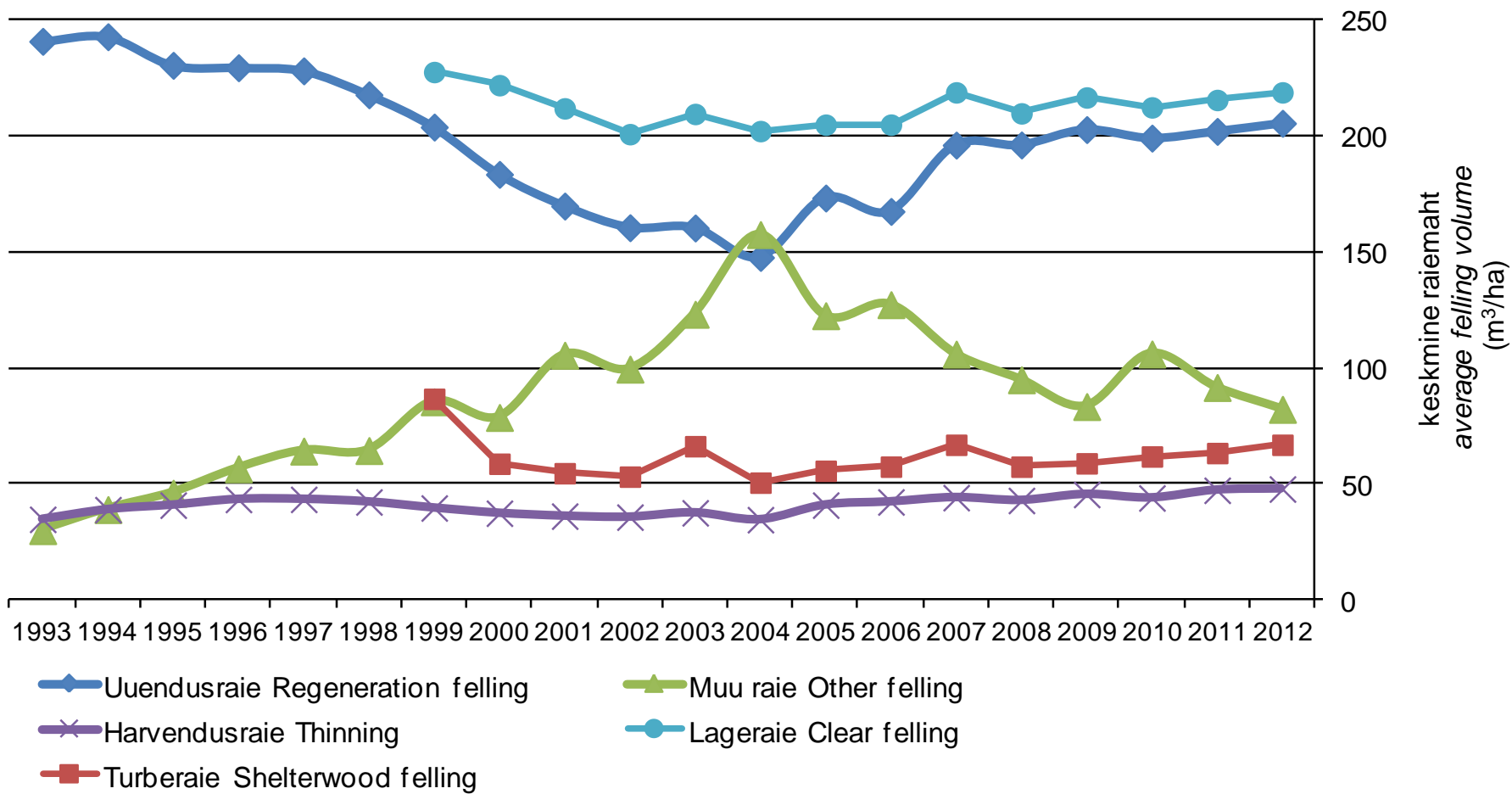
Joonis 3.3.3.1 Keskmise raiemaht hektari kohta aastail 1993–2012 (m³/ha)
